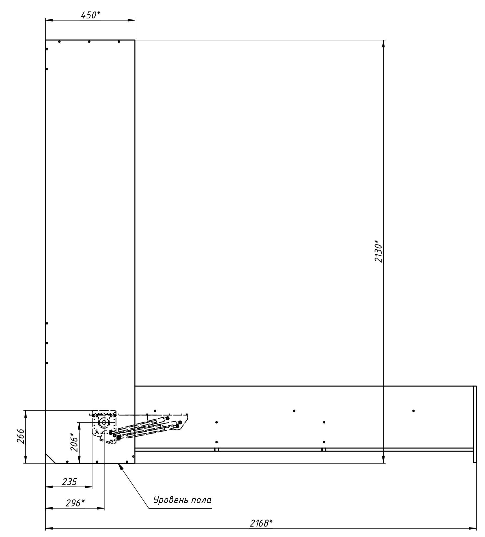
Изображена кровать в раскрытом положении
